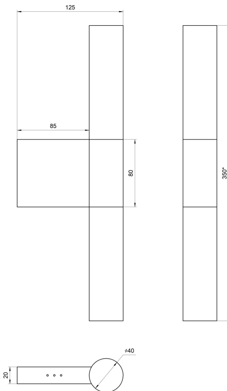
Рис.1 Внешний вид «Указатель лифтовой» НШЕК.468232.207
